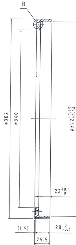
A-A断面図
