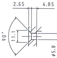
B部詳細図 (1:2)
