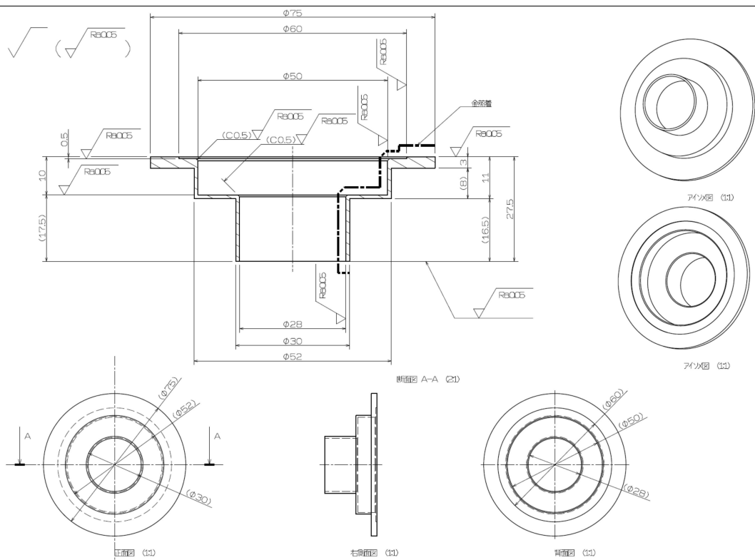
図 2.2.2-5 2 step A2 型 (F2-A2)
