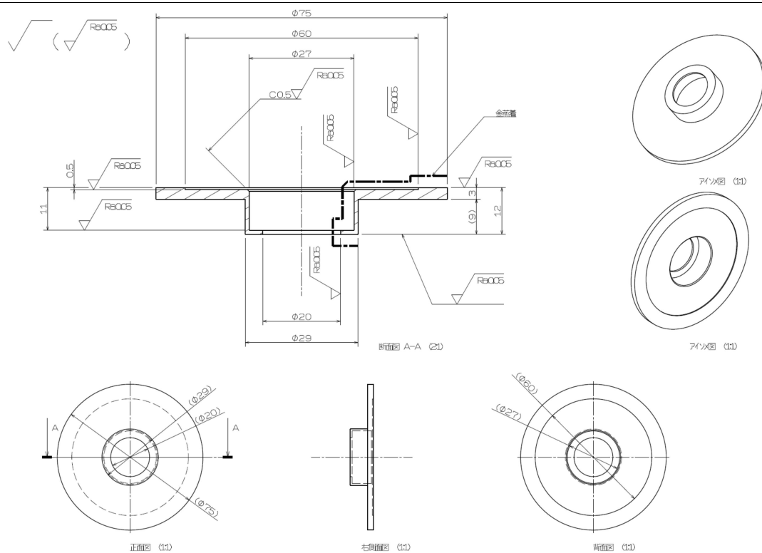
图 2.2.2-1 1 step A 型 (F1-A)
