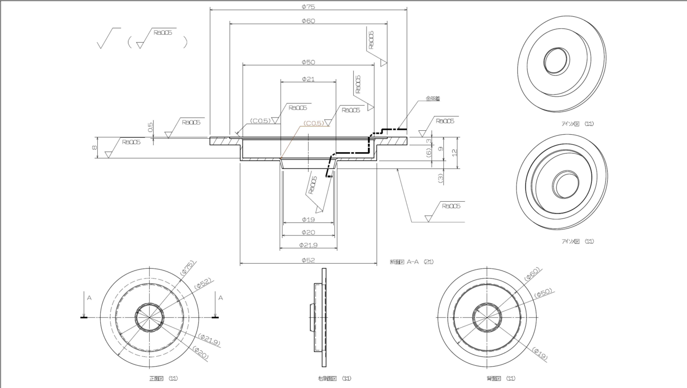
图 2.2.2-4 2 step B 型 (F2-B)
