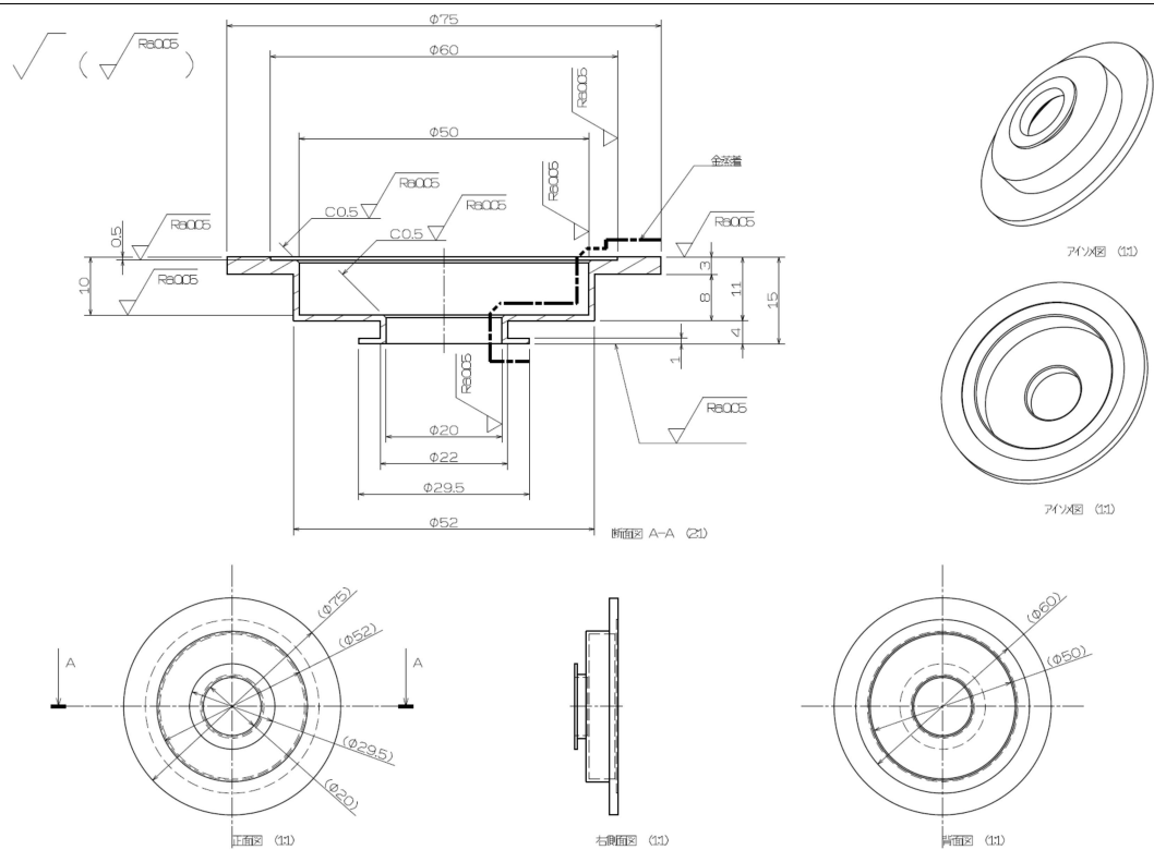
图 2.2.1-4 2 step B 型 (T2-B)
