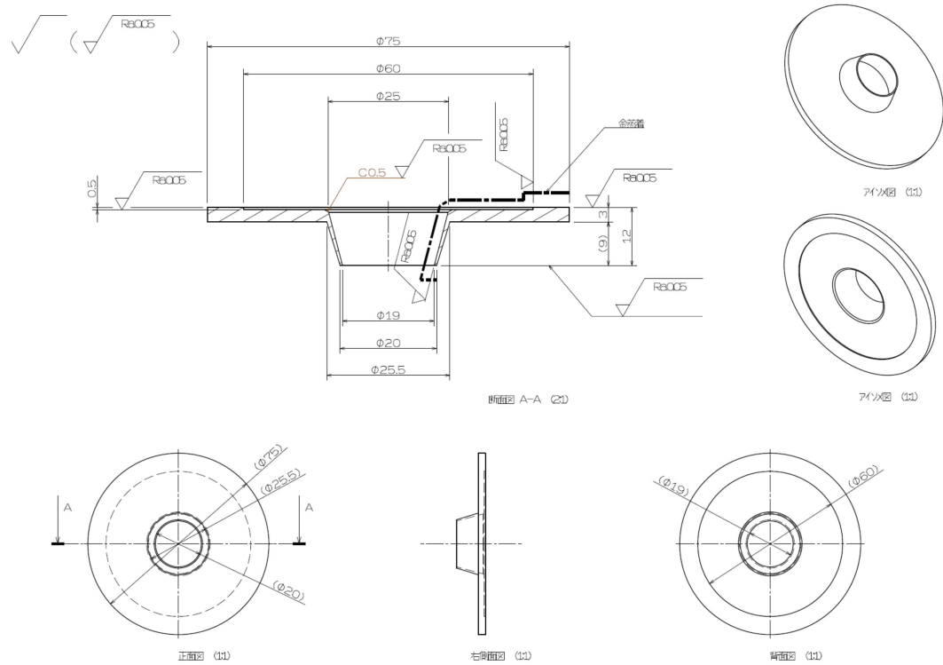
图 2.2.2-2 1 step B 型 (F1-B)
