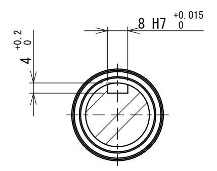
断面図 A-A
